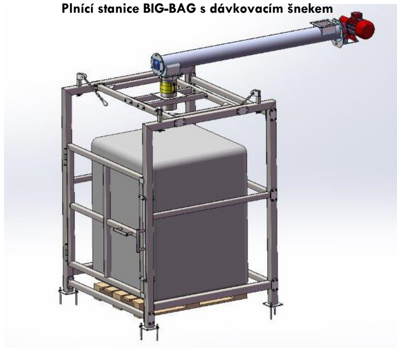
Plnicí stanice BIG-BAG s navažovací aparaturou
