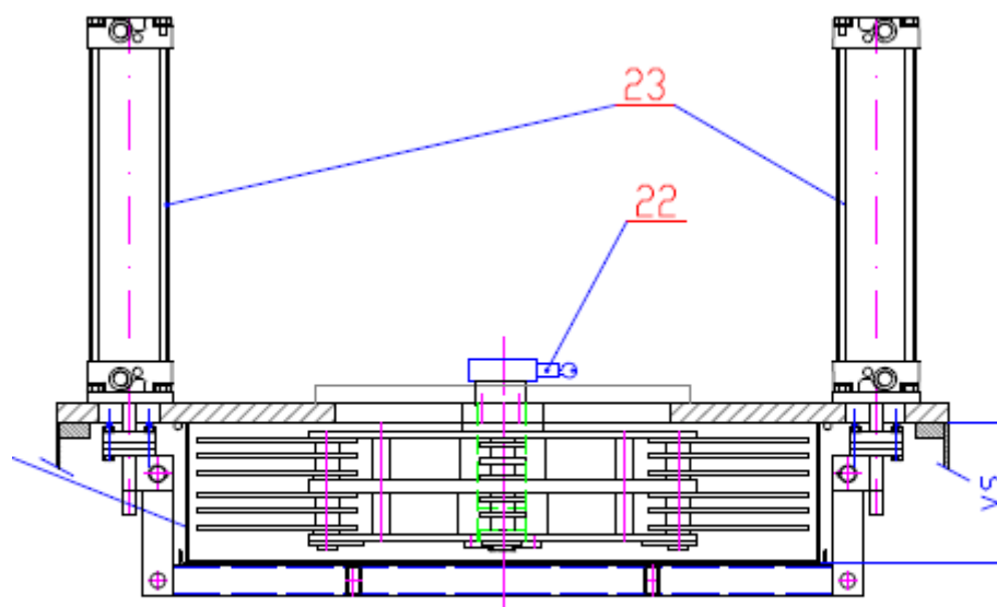
Pneumatické ovládání síta
