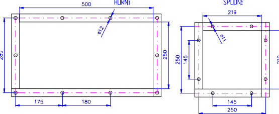
PŘIPOJOVACÍ ROZMĚRY PŘÍRUBY
